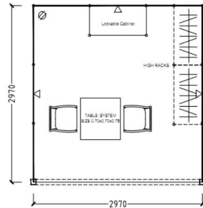
LAY-OUT PLAN
