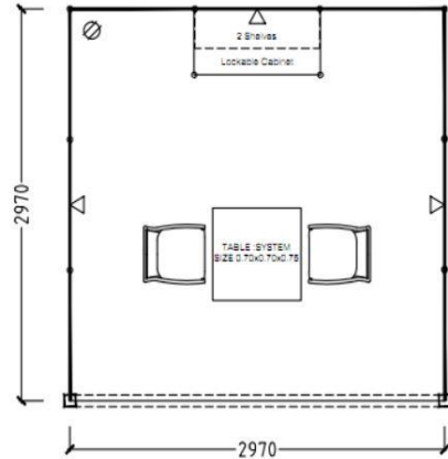
LAY-OUT PLAN
